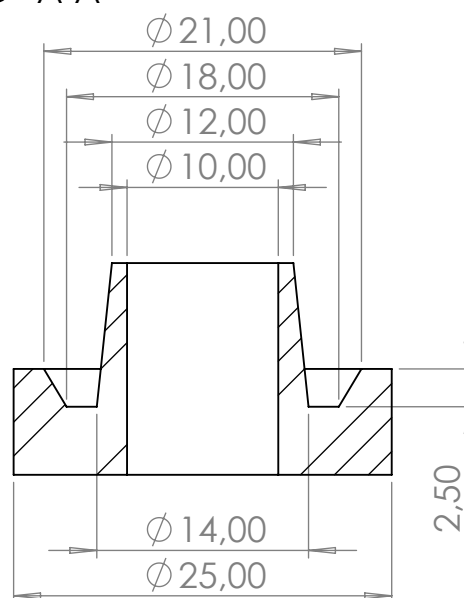
SEÇÃO B-B
